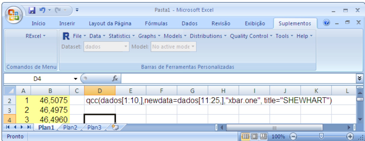
Figura 7. RExcel com os comandos para geração da Fase I e II do gráfico de controle tipo Shewhart para a média
