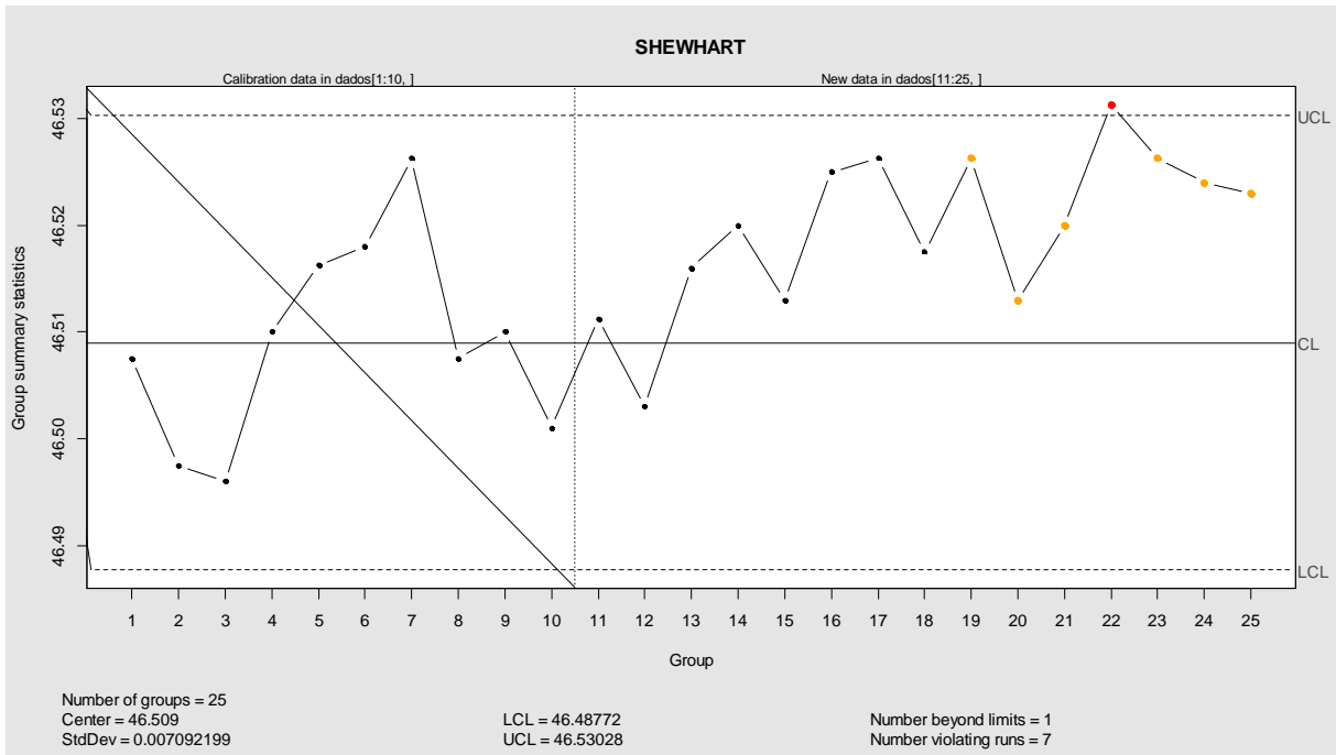
Figura 6. Gráfico de controle Shewhart para a média do processo de usinagem (fase de diagnóstico e monitoramento)
