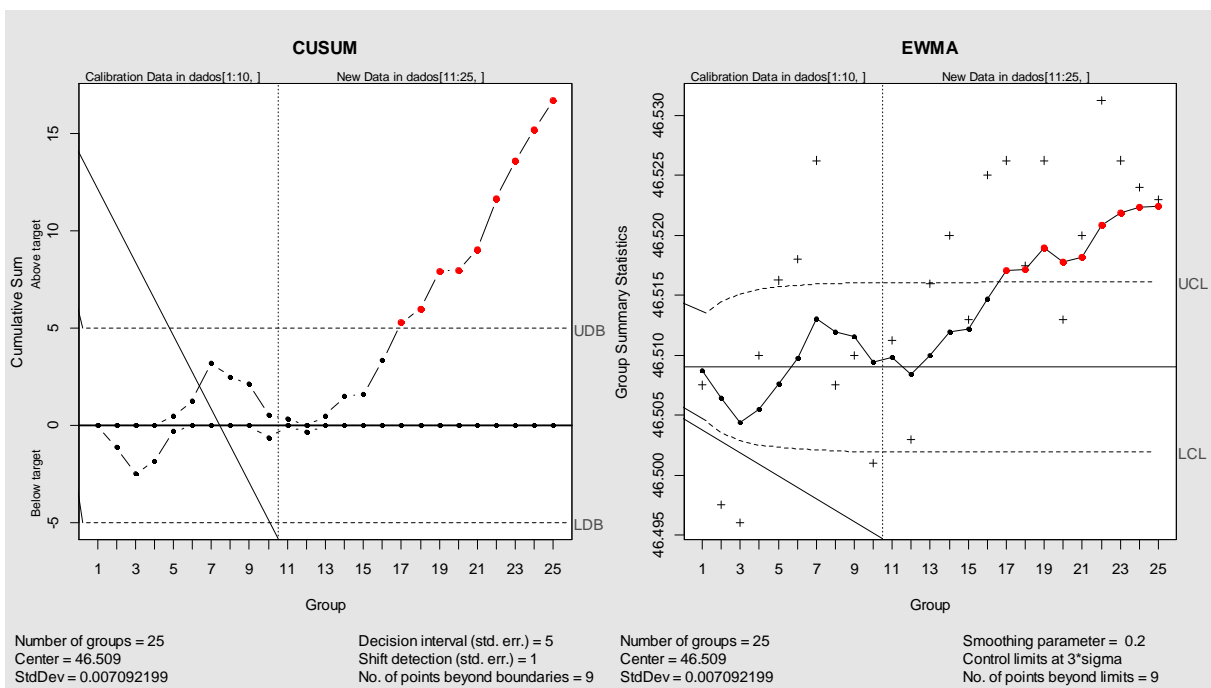
Figura 9. Fase de diagnóstico e monitoramento dos gráficos de controle CUSUM (esquerda) e EWMA (direita)
